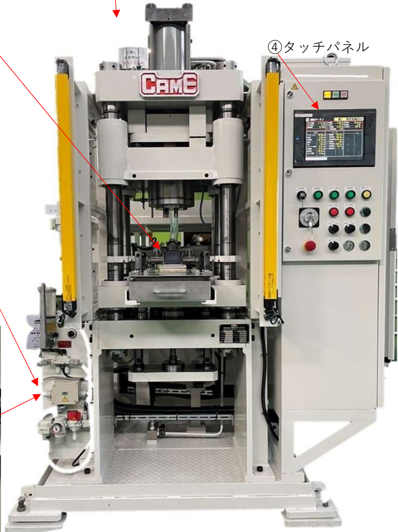
①②③省エネ・省スペース・ 静音性に優れた油圧ユニ ット(本体スペースに収納)
